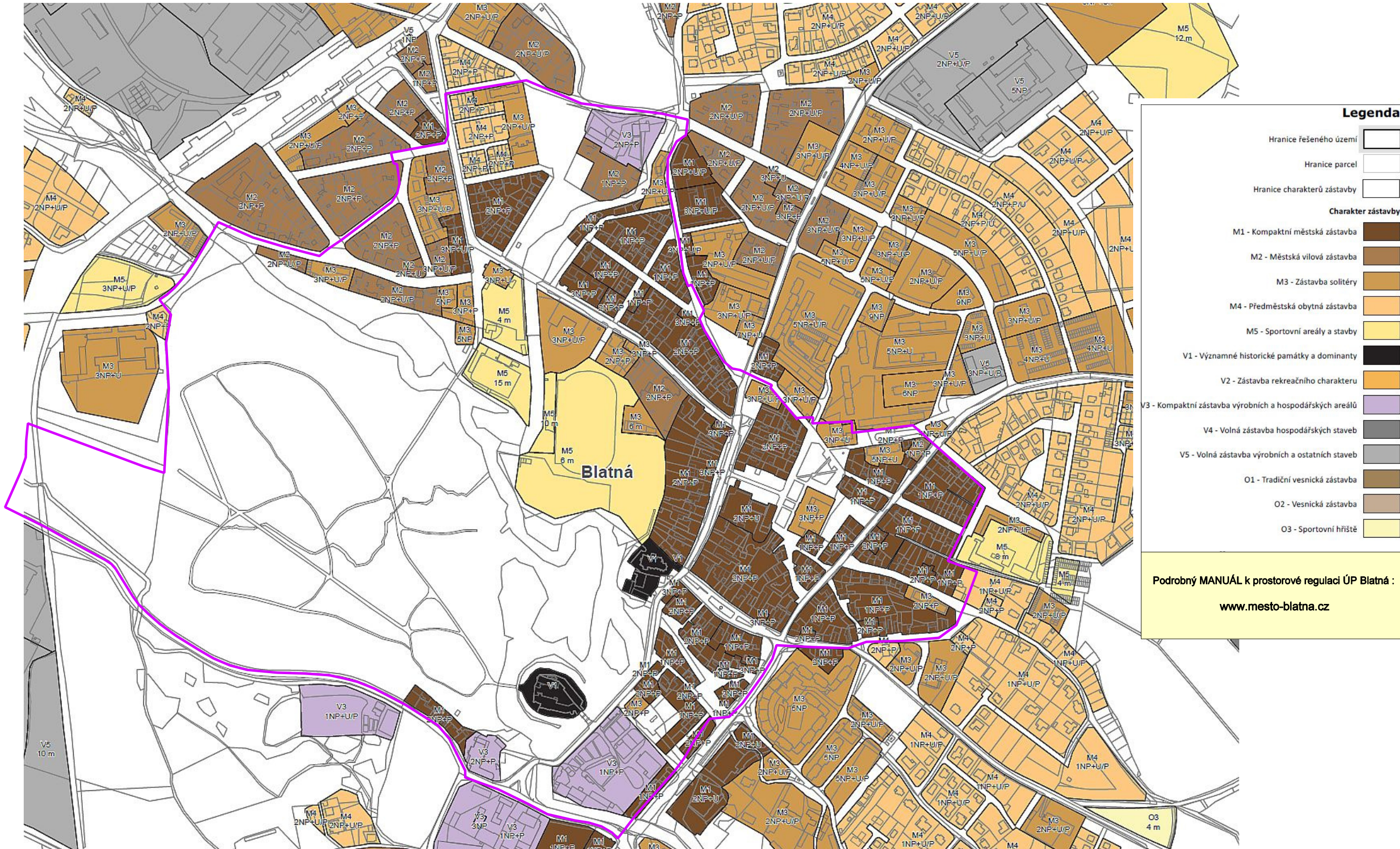
PROSTOROVÁ REGULACE - ZMENŠENÝ VÝŘEZ SNÍMKU HLAVNÍHO VÝKRESU ÚZEMNÍHO PLÁNU HRANICE MPZ BLATNÁ
